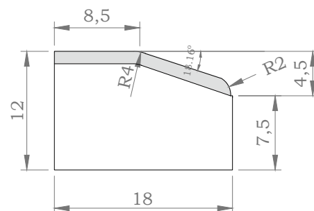
PRESEK A-A
