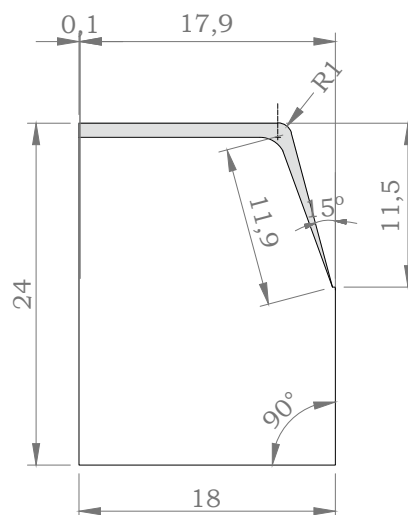
PRESEK A-A
