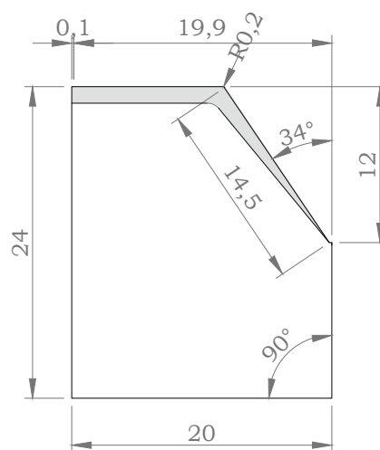
PRESEK A-A
