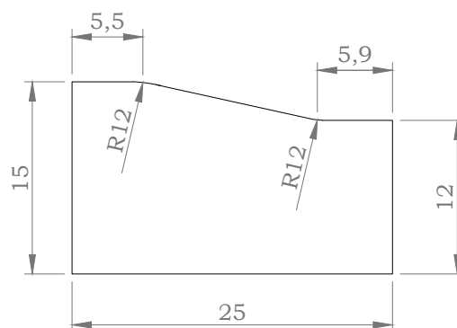
PRESEK A-A
