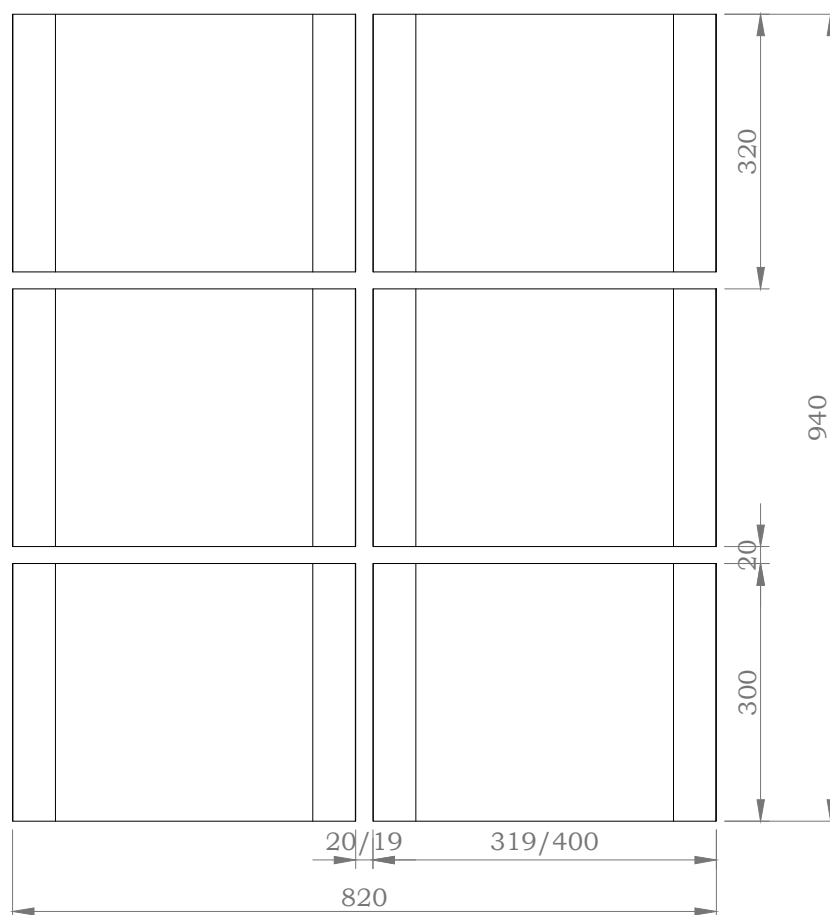
DIMENZIJE MODULA
