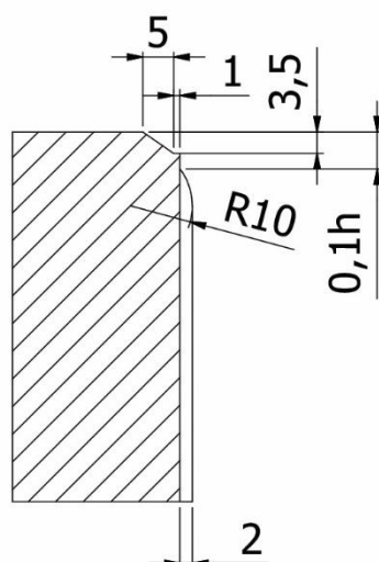
A-A ( 1 : 1 )
