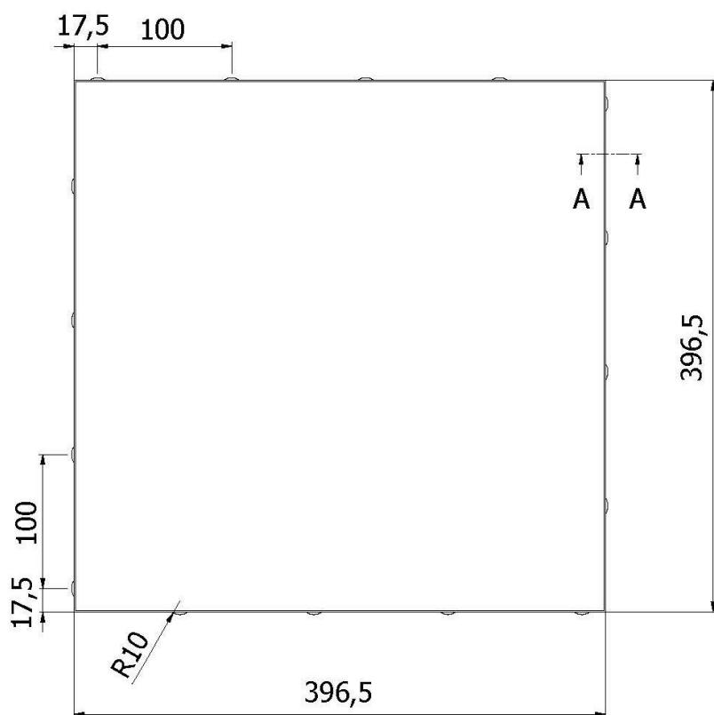
A-A ( 1 : 1 )
