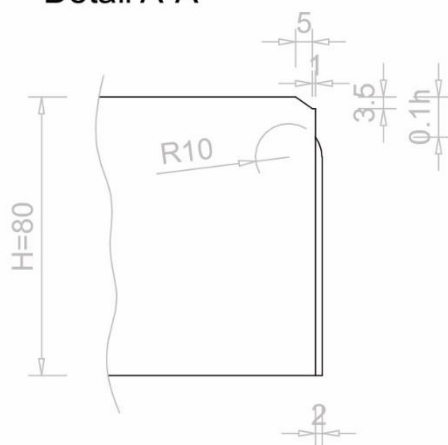
Detail A-A
