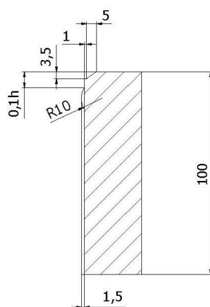
A-A (1-1)
