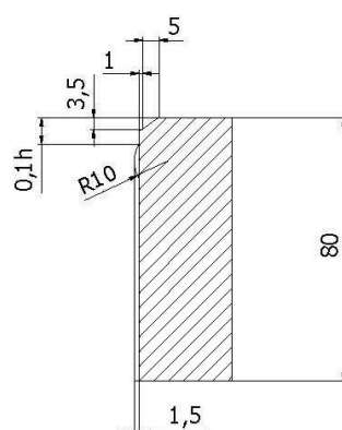
A-A (1-1)
