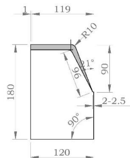
PRESEK A-A
