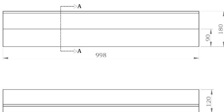
DIMENZIJE MODULA
