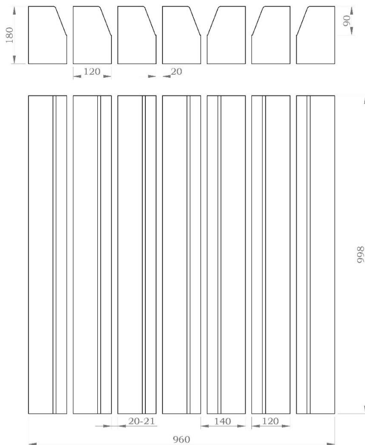
DIMENZIJE MODULA
