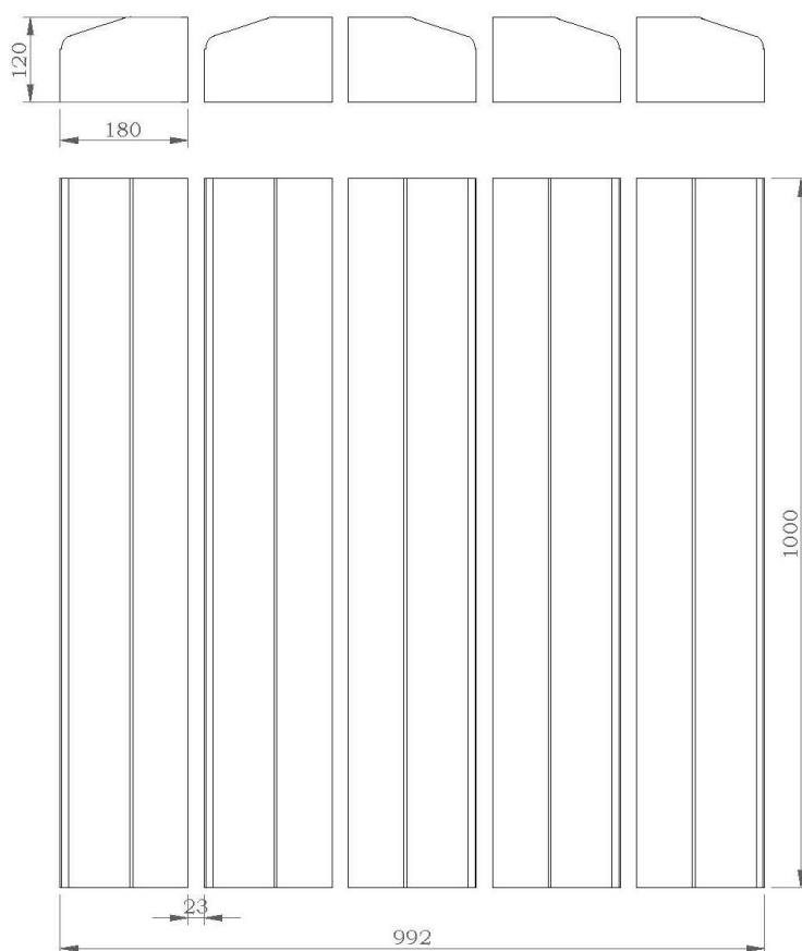
DIMENZIJE MODULA
