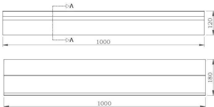
DIMENZIJE MODULA
