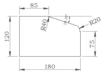
PRESEK A-A
