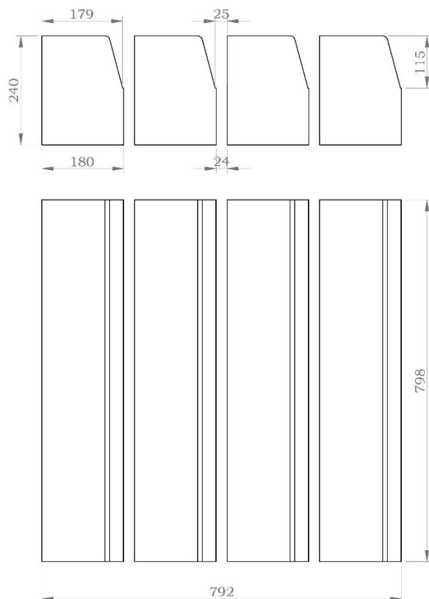
DIMENZIJE MODULA
