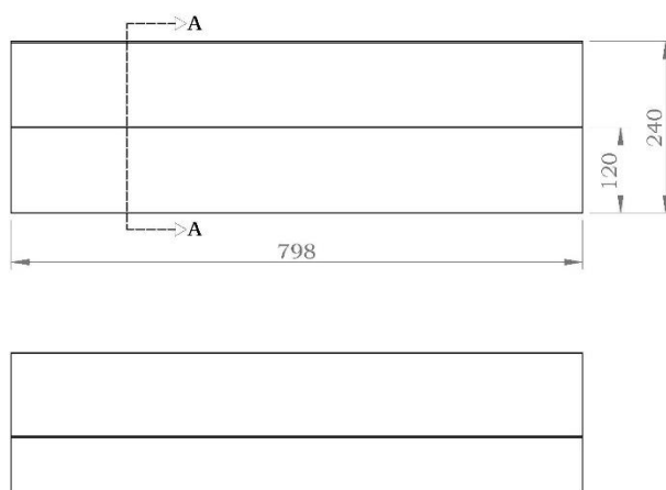
DIMENZIJE MODULA
