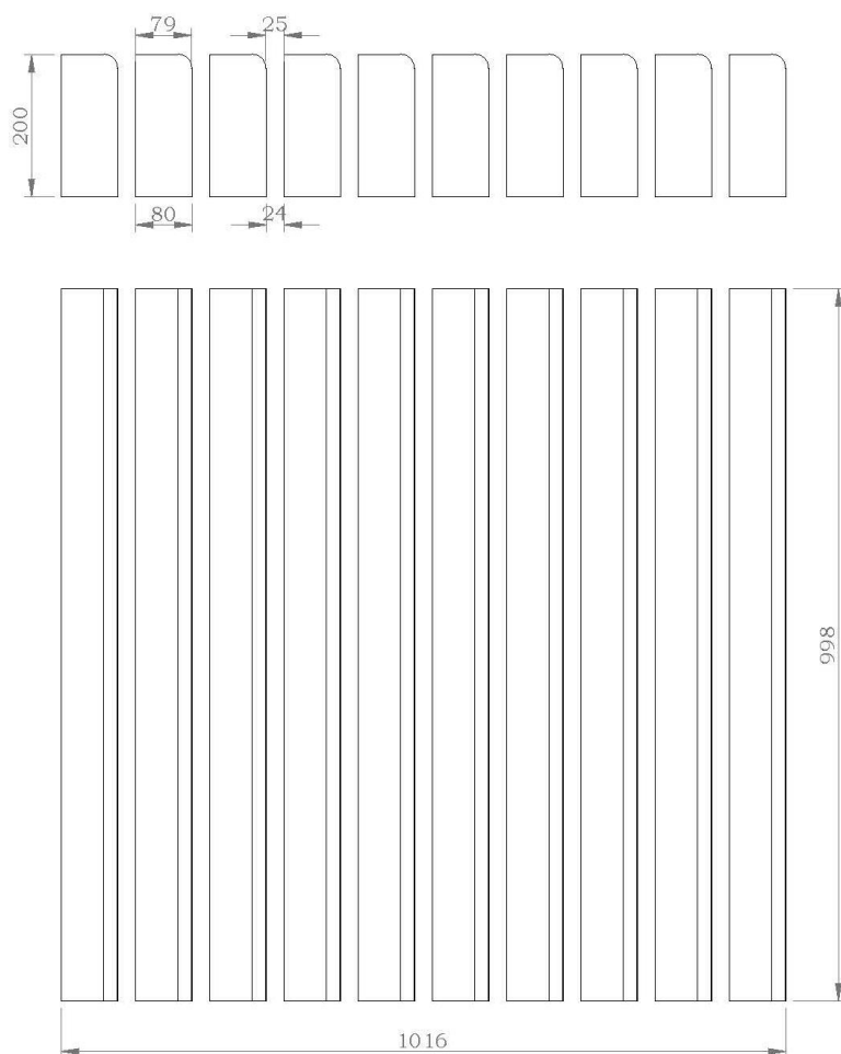
DIMENZIJE MODULA
