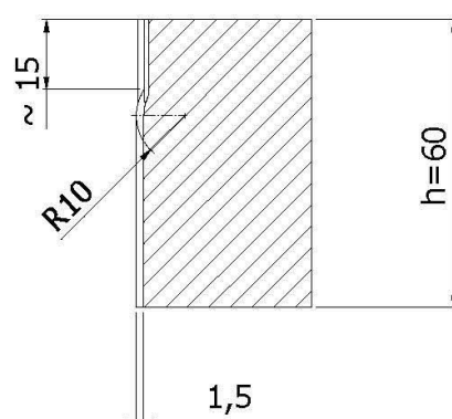
B-B ( 1 : 1 )
