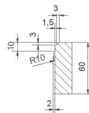
Presek A-A (1:1)
