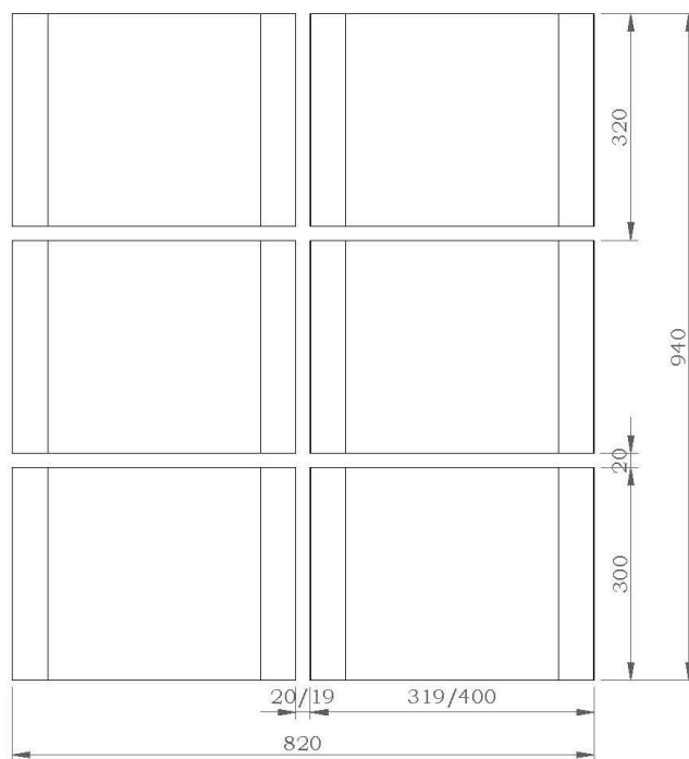
DIMENZIJE MODULA
